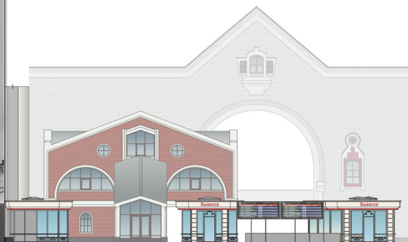
Развертка В-В М 1:100
