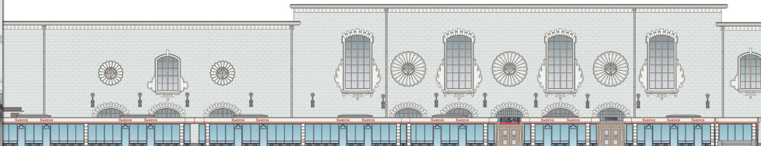
Развертка В-В М 1:100
