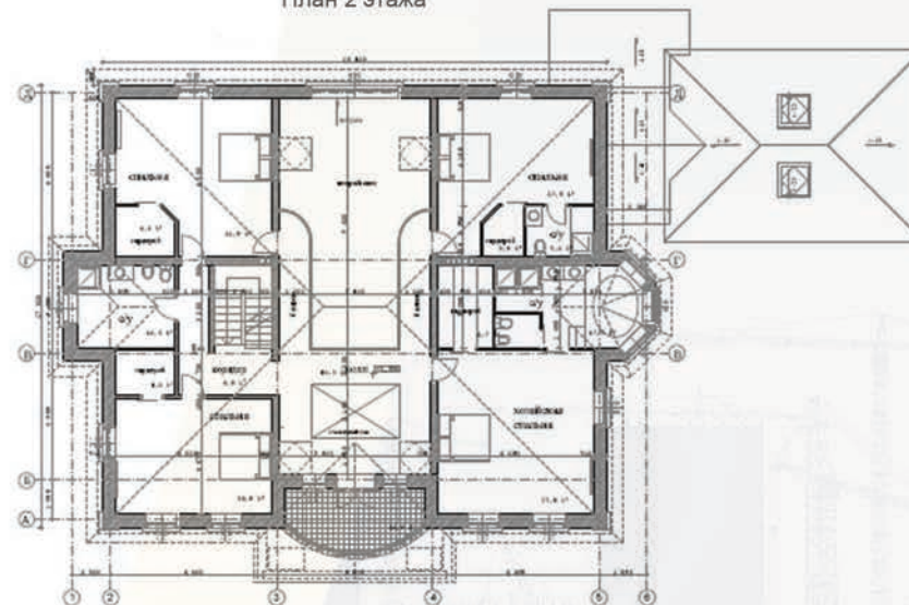
План 2 этажа
